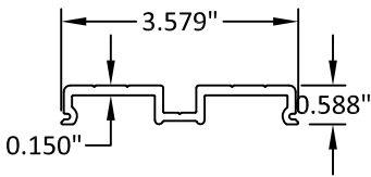
5 1/4" CORNER SLEEVE E9-7049
