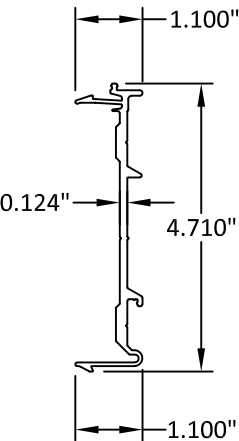
5 1/4" INTERLOCKING CLIP E9-7003
