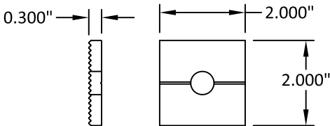
LOCK WASHER E1-3908
